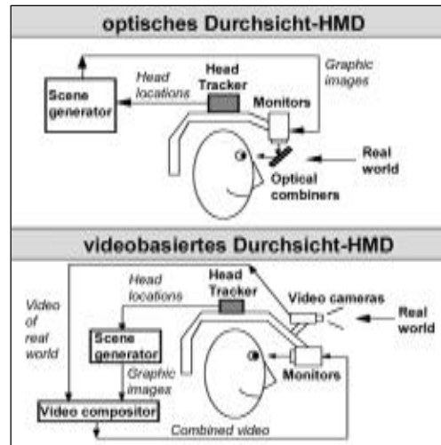
Bild 1: Datenbrillen funktionieren im optischen Durchsichtmodus (reale Welt ist durch halbdurchlässige Spiegel oder Prismen sichtbar, zusätzlich werden virtuelle Objekte eingeblendet) oder im Video-Durchsichtmodus (Kamerabild wird mit virtuellen Objekten angereichert) [2]
